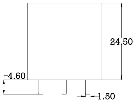
图 3 模组外观尺寸图
